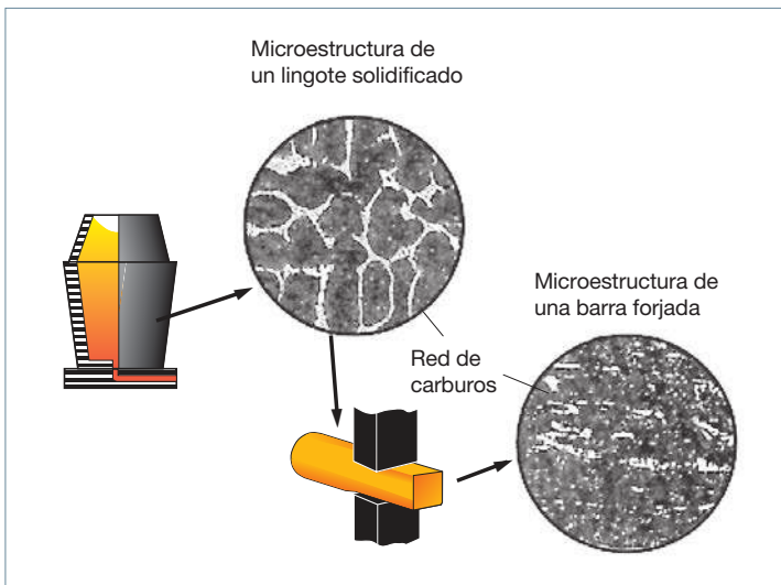
Fig. 5. Rotura de la red de carburos durante la operación de forjado en caliente de lingotes de acero.
