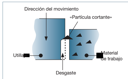
Fig. 2. Representación esquemática de desgaste abrasivo.
