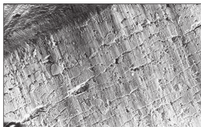
Foto 2. Fotografía SEM de un punzón realizado con material D2 fuera de servicio a causa del desgaste adhesivo (material de trabajo, acero inoxidable austenítico).
