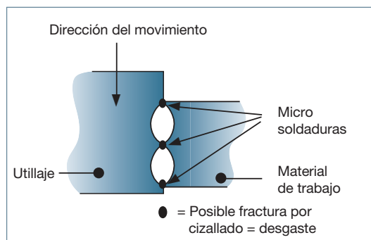
Fig. 4. Representación esquemática de desgaste adhesivo.
