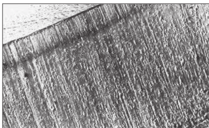
Foto 1. Fotografía SEM de un punzón realizado con material D2 fuera de servicio a causa del desgaste abrasivo (material de trabajo acero 1% C a 46 HRC).
