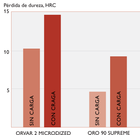
Fig. 1. Pérdida de dureza al cabo de 24 horas a 600°C durante la compresión
